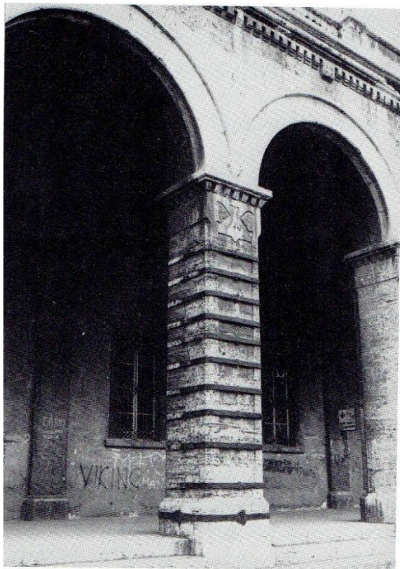
Palazzo della Provincia di Perugia. Cerchiatura di un pilastro di sezione quadra ta, contro lo schiacciamento.
