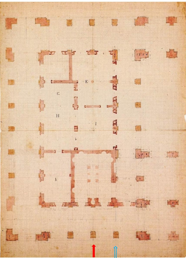
Palazzo della Provincia di Perugia. Veduta d'insieme con alcuni dei pilastri cerchiati contro lo schiacciamento cubico.
